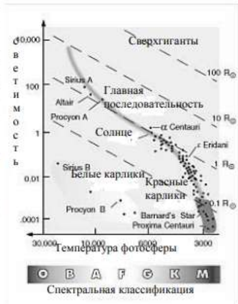
Рис.14 Диаграмма Герцишпрунга-Рассела
