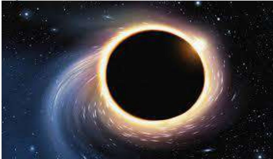
Рис. 1 – Черная дыра
