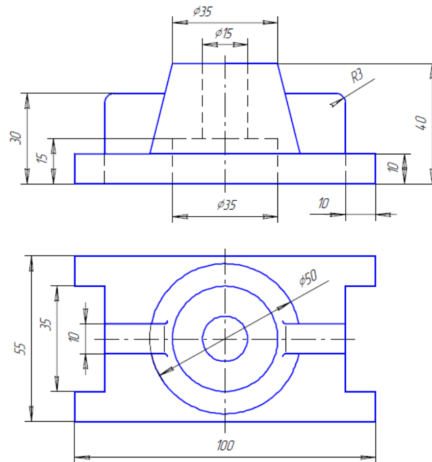
Стойка Вариант 2
