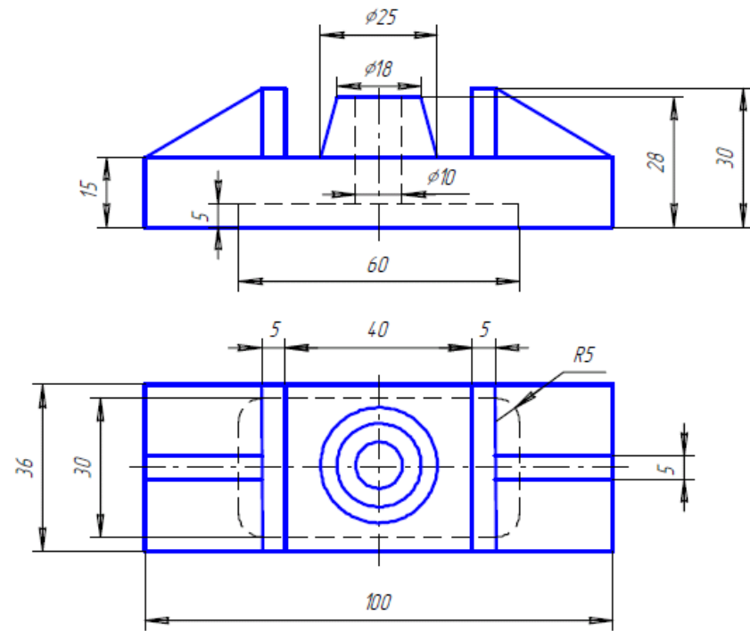
Опора Вариант 10
