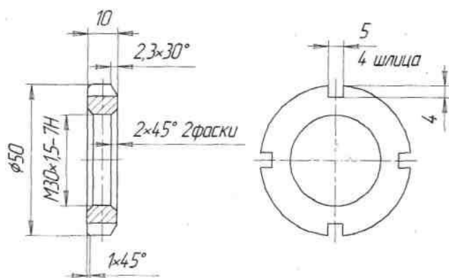
Рис. 3 Гайка
