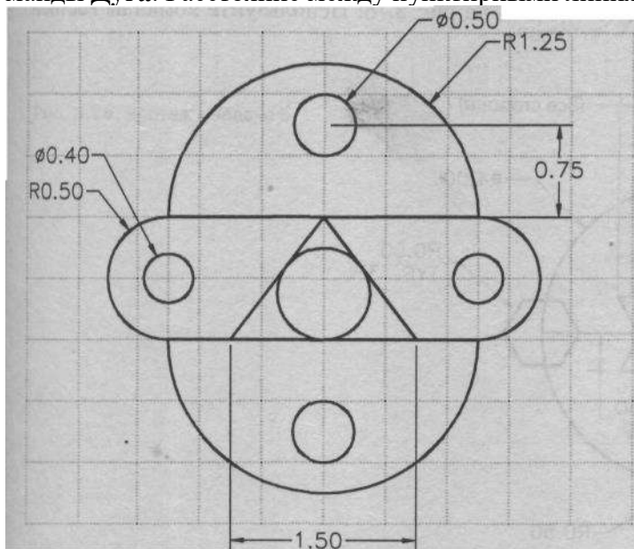
Рисунок 3.16. Чертеж к задаче 2
