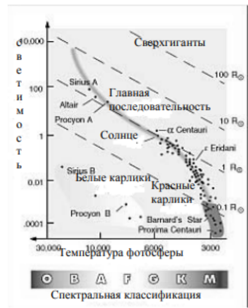
Рис.14 Диаграмма Герцигунга-Рассела
