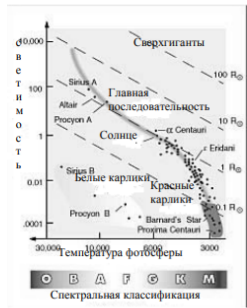
Рис.14 Диаграмма Герцигунга-Рассела
