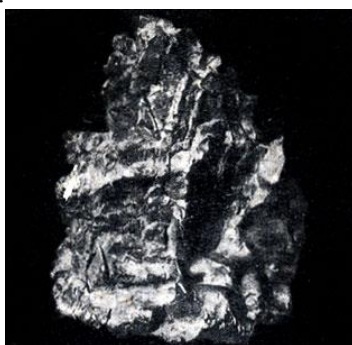
Рис. 59. Железный метеорит
