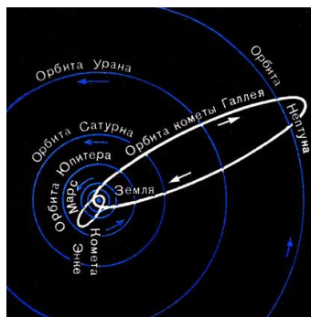
Рис. 61. Орбиты комет Галлея и Энке
