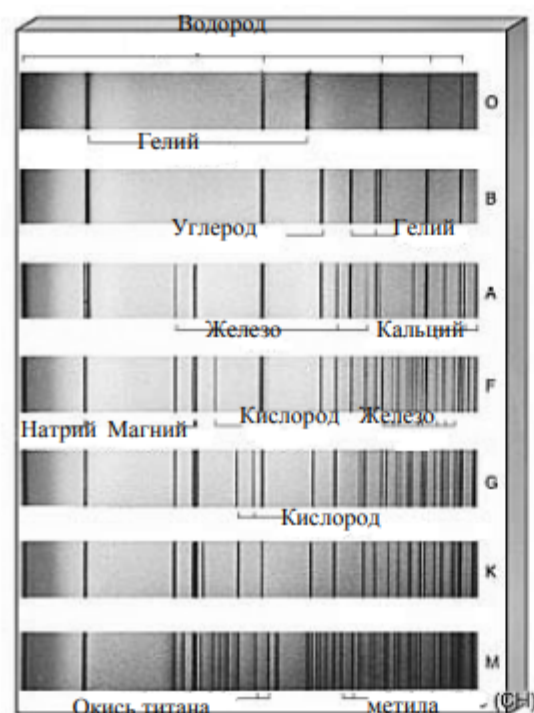
Рис. 13 Спектры
